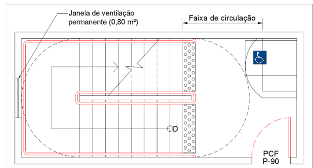
Figura 7: Escada enclausurada protegida
