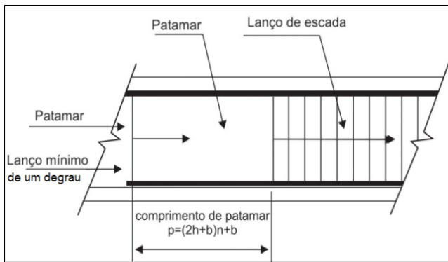
Figura 6: Lanço mínimo e comprimento de patamar
