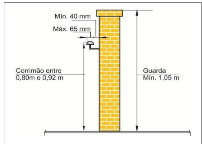
Figura 15: Dimensões de guardas e corrimãos
