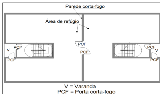
Figura 18: Desenho esquemático da área de refúgio
