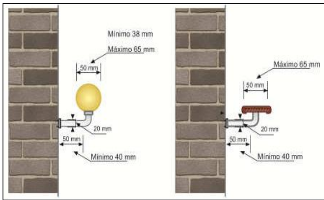
Figura 16: Pormenores de corrimãos
