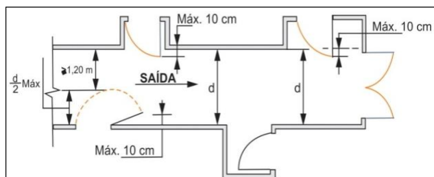
Figura 2: Abertura das portas no sentido de saída
