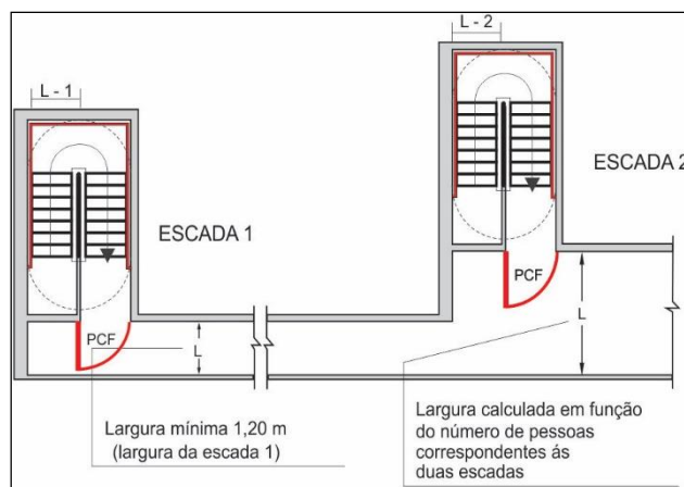
Figura 19: Dimensionamento de corredores de descarga
