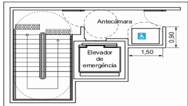
Figura 9: Escada enclausurada à prova de fumaça, com área para pessoas com deficiência.
