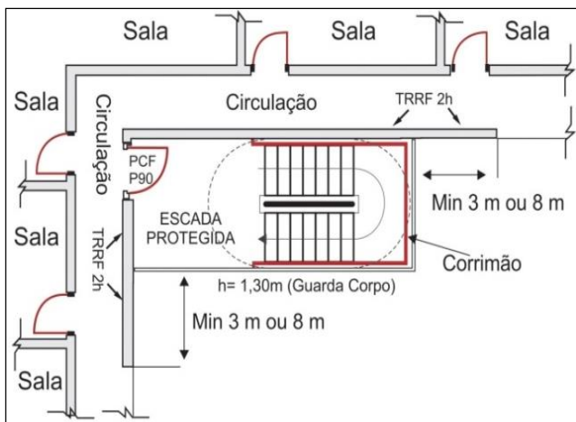
Figura 14: Escada aberta externa
