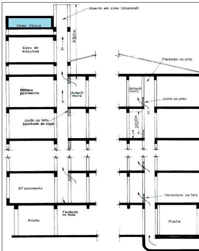
Figura 11: Exemplo de dutos de ventilação (corte AB e corte CD)
