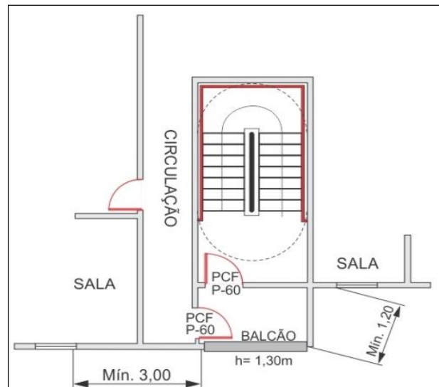
Figura 12: Escada enclausurada do tipo PF ventilada por balcão
