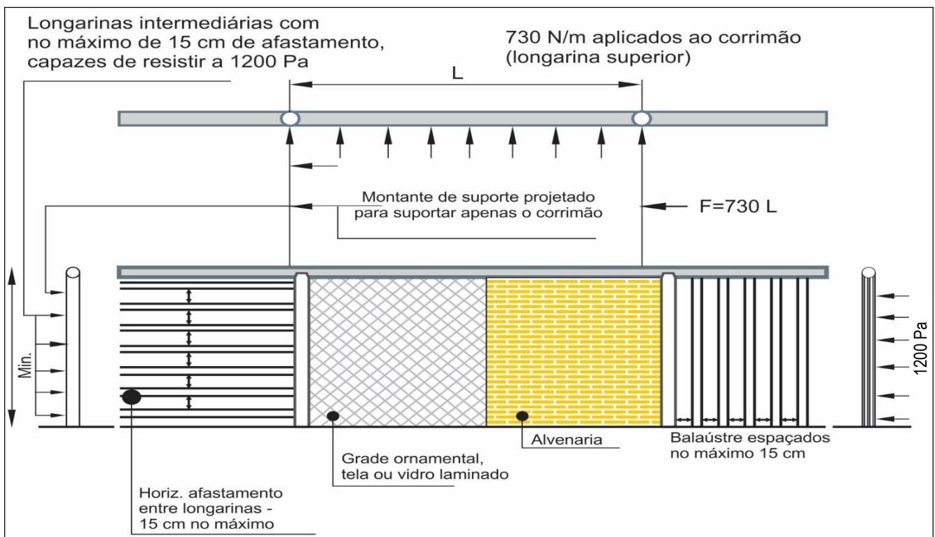
Figura 17: Pormenores construtivos da instalação de guardas e as cargas a que elas devem resistir
