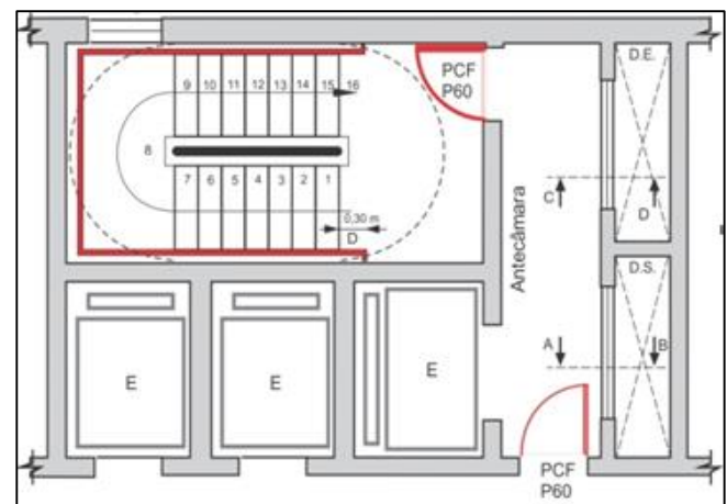
Figura 10: Escada enclausurada à prova de fumaça (demonstração dos dutos)
