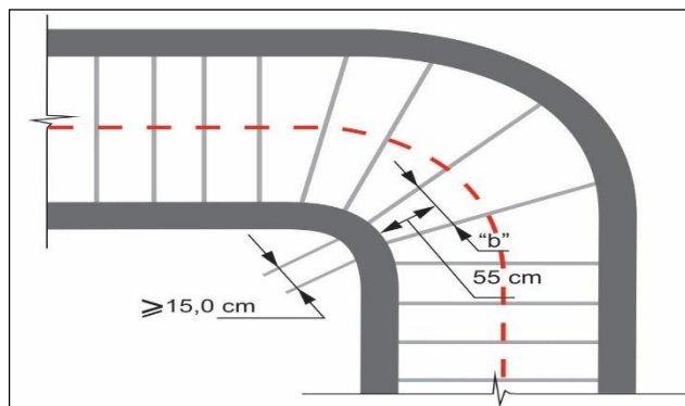
Figura 5: Escada com patamar em leque, degraus balanceados, permitida para acesso a mezaninos e áreas restritas
