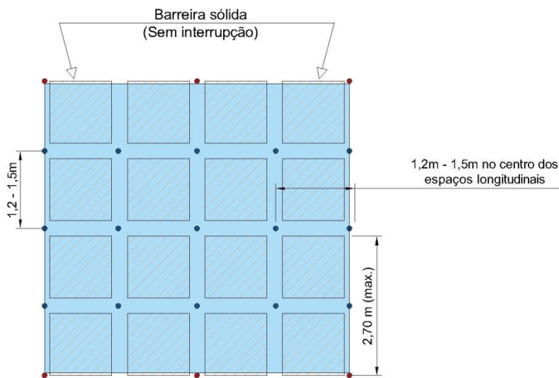
Planta baixa
